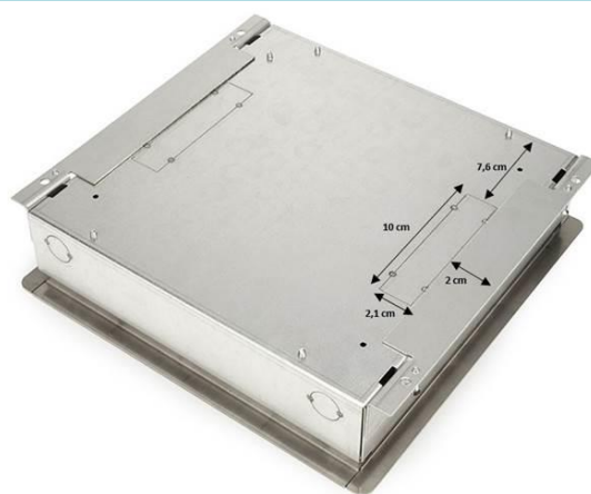
Standaard sparring voor kabelinvoer vanaf de onderzijde
